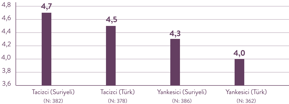
ŞEKİL 44: ŞİDDET ONAYI
