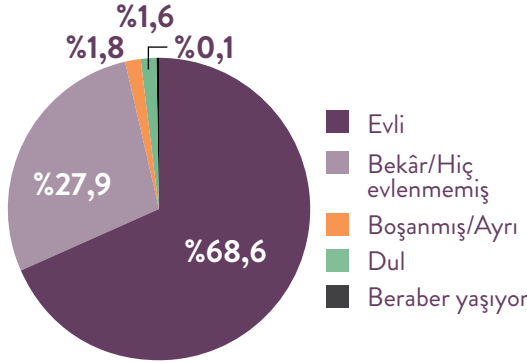
ŞEKİL 7: MEDENİ DURUM
