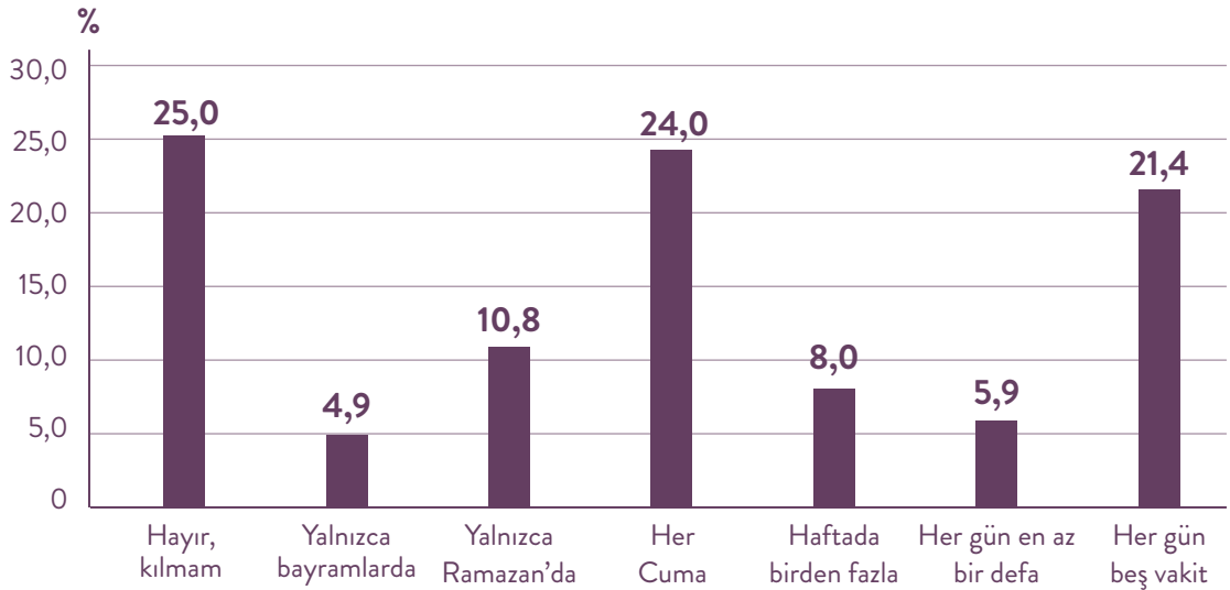
ŞEKİL 9: İBADET SIKLIĞI
