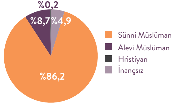
ŞEKİL 8: DİNİ İNANÇ
